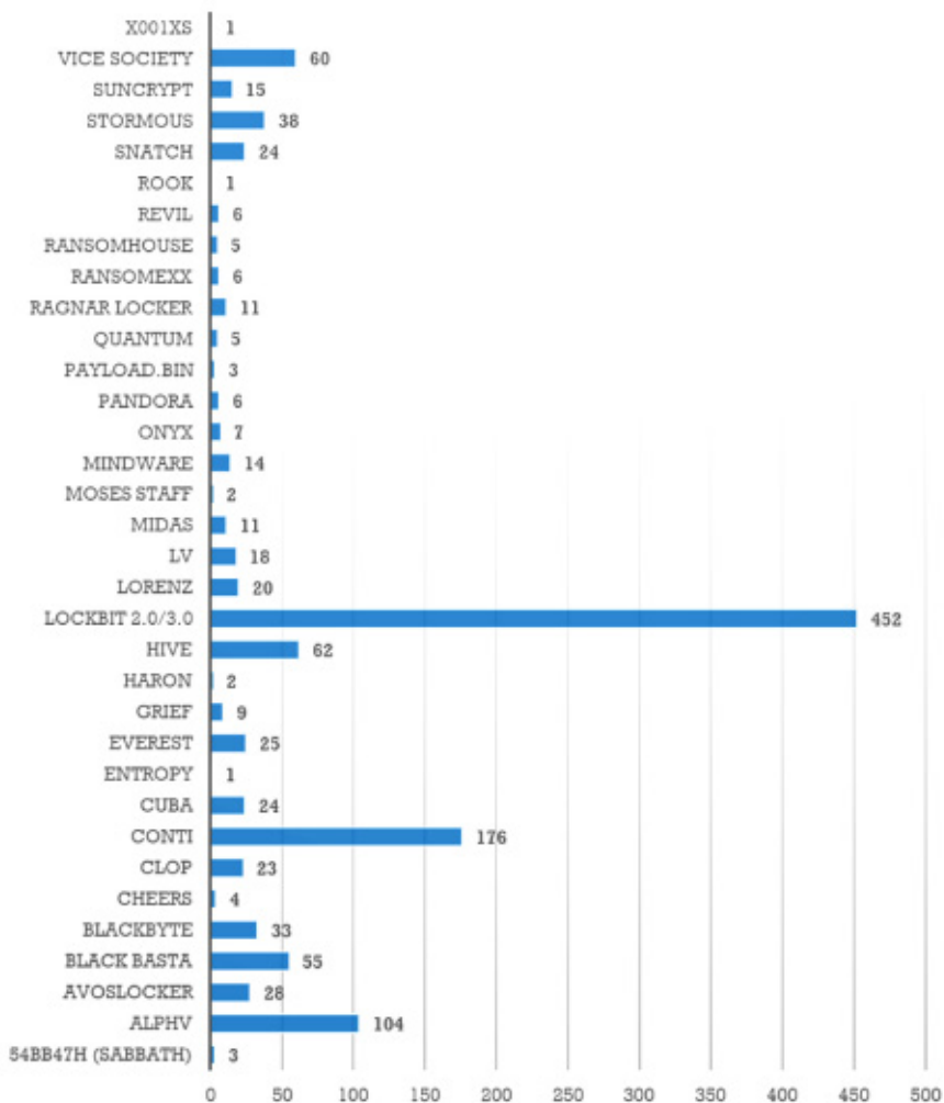
勒索软件攻击活动(2022年1月—6月)
